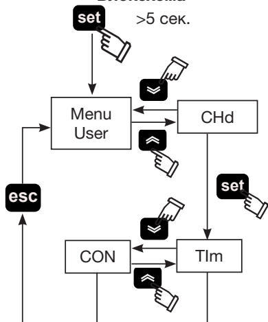
Блоксхема
